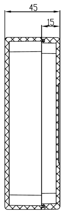
A-A
