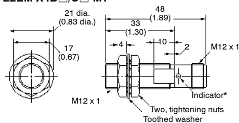
E2EM-X4B□/C□-M1
