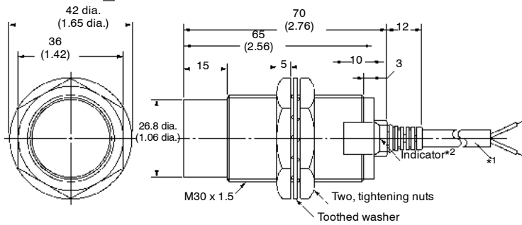
E2EM-X30MX□
