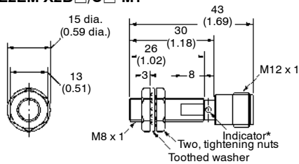
E2EM-X2B□/C□-M1
