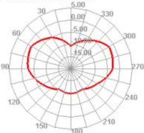
3300.000MHz E2
