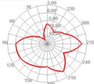
2100.000MHz E2
