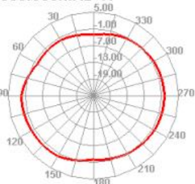
4800.000MHz H
