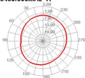
3435.000MHz H
