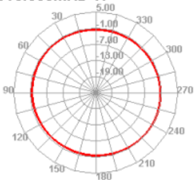
960.000MHz H
