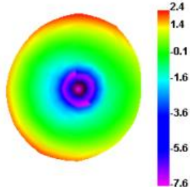
3705.000MHz E1
