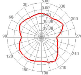
900.000MHz E1
