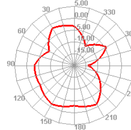
960.000MHz E1
