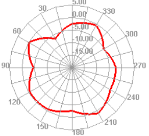
900.000MHz E2
