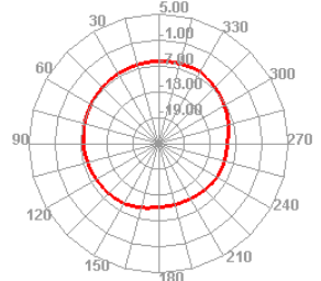
1700.000MHz E2
