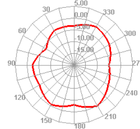
960.000MHz E2
