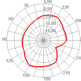
820.000MHz E1
