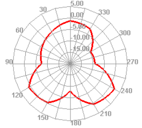
1700.000MHz E2
