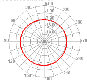
1800.000MHz E2
