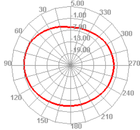
820.000MHz E2
