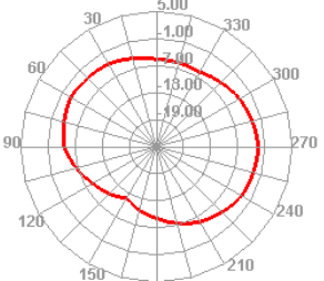
900.000MHz E2
