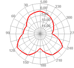
1700.000MHz E1
