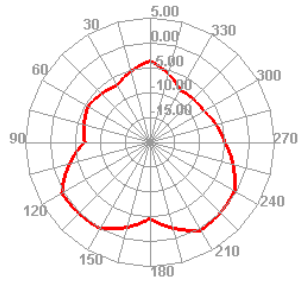
1800.000MHz E1
