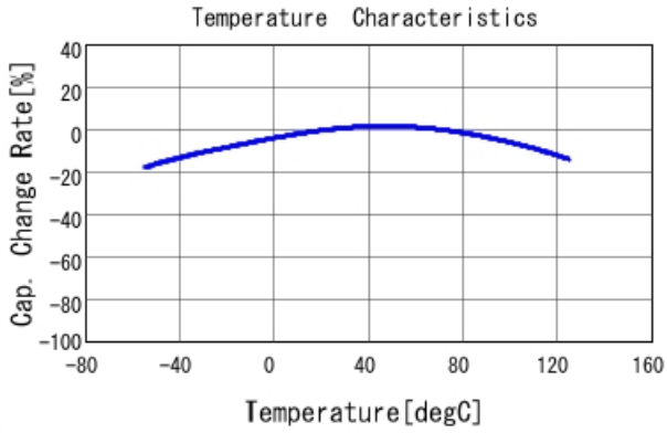
■ GCM155C71A105KE38 C-Temp. capchange, DCO. 0V, ACO. 2V rm
