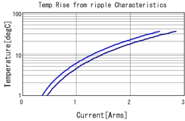
■ GCM155C71A105KE38 Temp. rise ■ 500kHz ■ 1MHz
