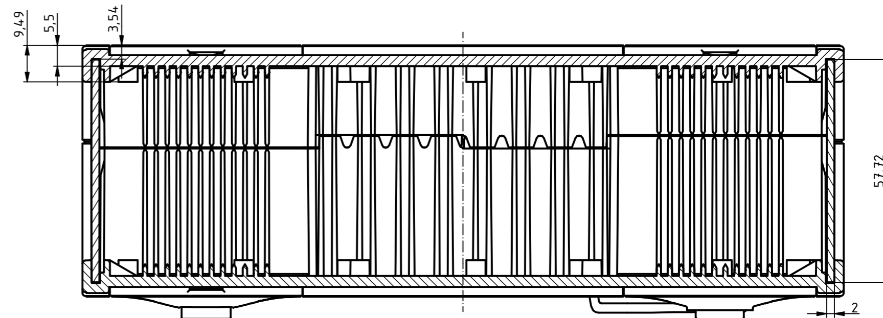
A-A (1:1)
