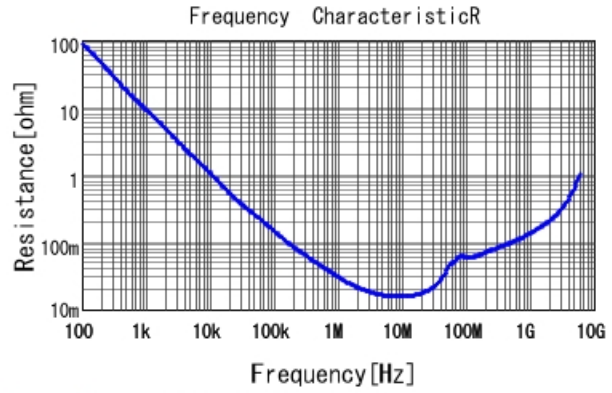
GRM155R61H104KE14 R DCOV, 25degC
