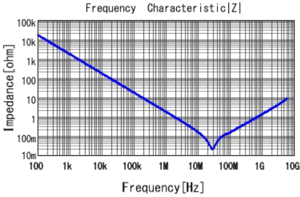
GRM155R61H104KE14 |Z| DCOV, 25degC
