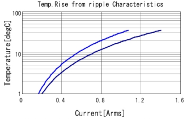
GRM155R61H104KE14 Temp. rise — 500kHz — 1MHz
