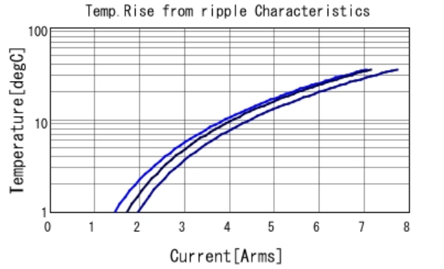
GRM32ER61A107ME20 Temp. rise — 50kHz — 200kHz
