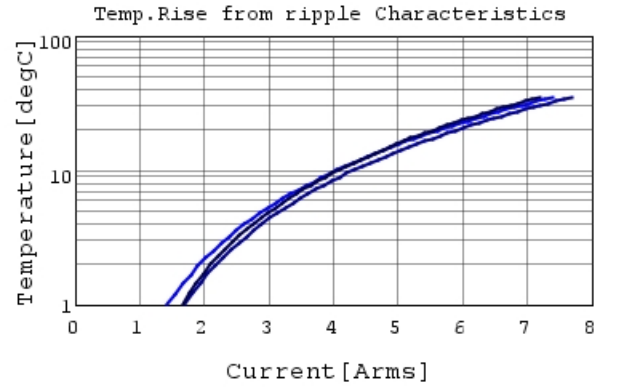
GRM21BR60J107ME15 Temp.rise — 50kHz
