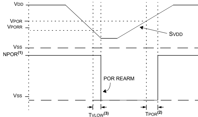
Figure 39-3. POR and POR Rearm with Slow Rising V_{DD}
