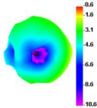
2400.000MHz E1
