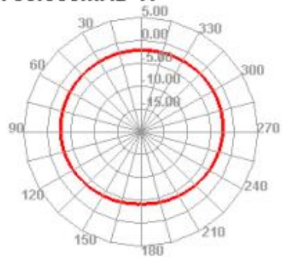
700.000MHz H
