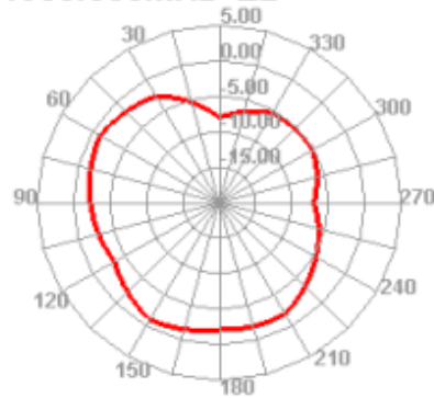
2100.000MHz H
