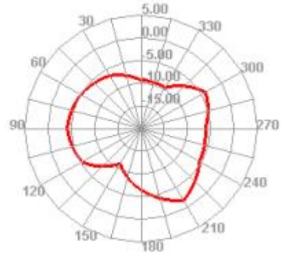
2400.000MHz E2
