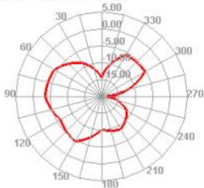
2500.000MHz E1
