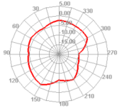
2300.000MHz H
