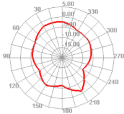
2300.000MHz
