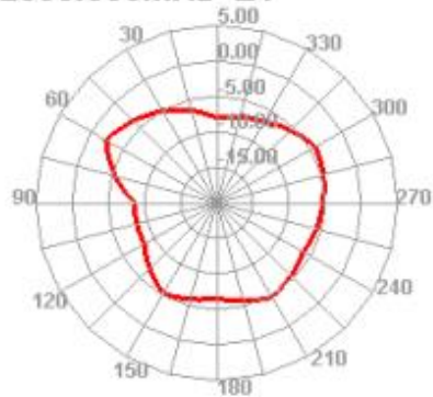
2300.000MHz E1
