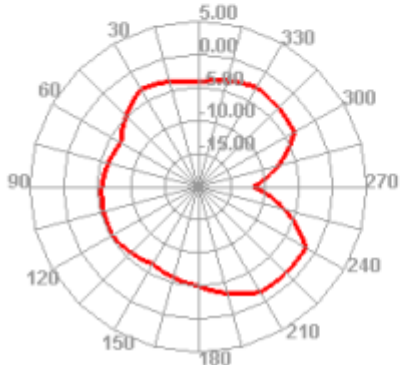
900.000MHz E1
