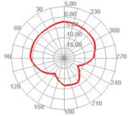
2400.000MHz H
