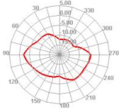
700.000MHz E1
