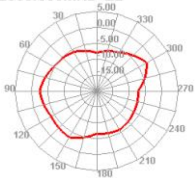
2300.000MHz E2
