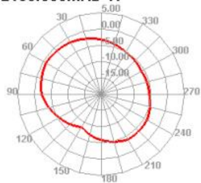
2100.000MHz H
