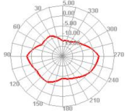
700.000MHz E2
