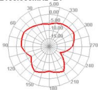
2100.000MHz E1
