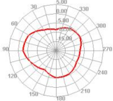
2300.000MHz H
