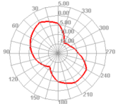
900.000MHz E2
