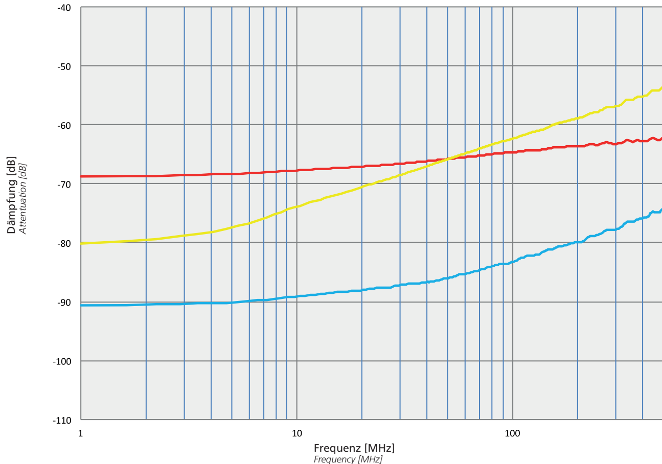
Schirmdämpfung Screen attenuation
