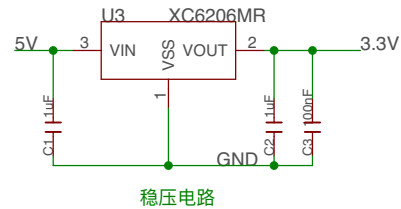
稳压电路
