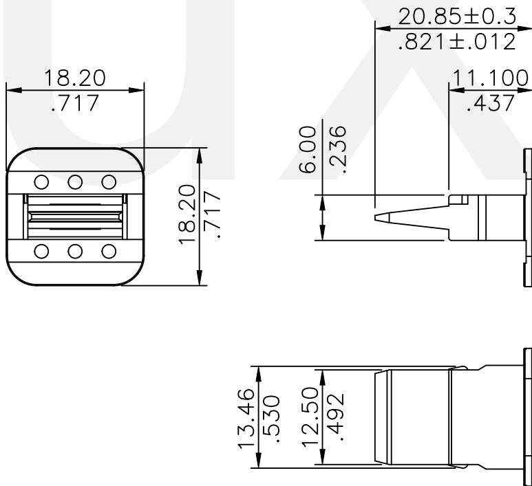
WEDGELOCK
