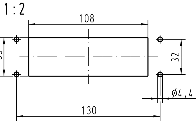
Montageausschnitt/ panel cut out
