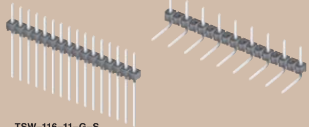
TSW-116-11-G-S
