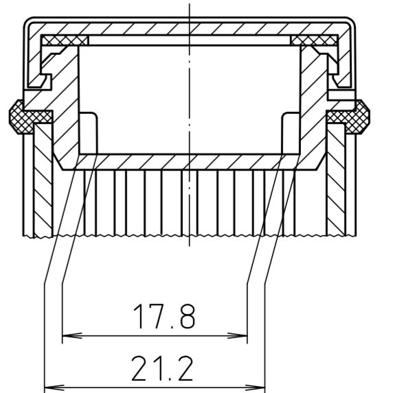
ABM 1000 AL
