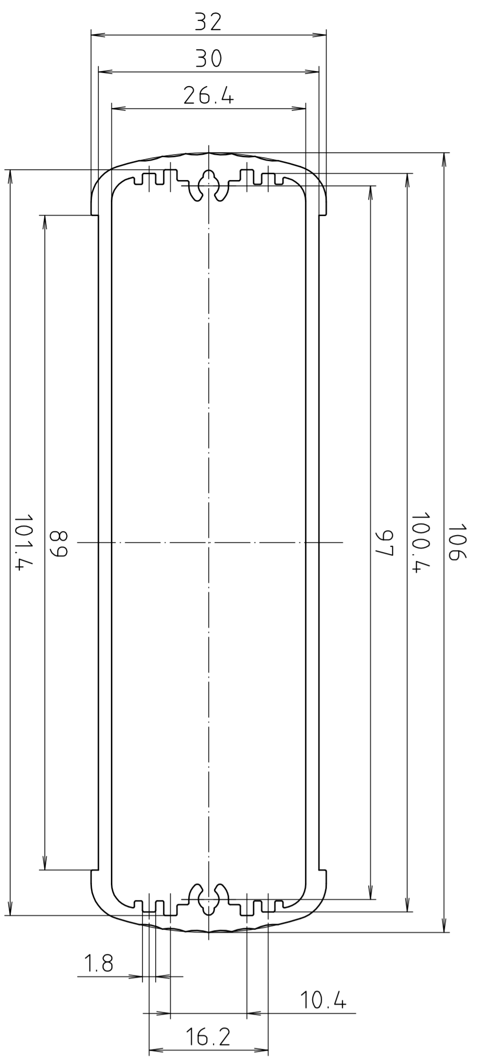
ABP 1000
