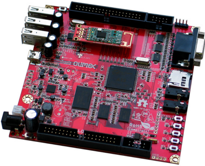
A13-OLinuXino-WIFI
