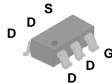
SOT-363 (SC-70-6)
