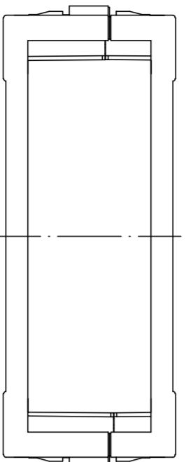
BO 32009 / BO 32009 L (Halbschale niedrig/hoch) BO 32009 / BO 32009 L (half shell low/high)
