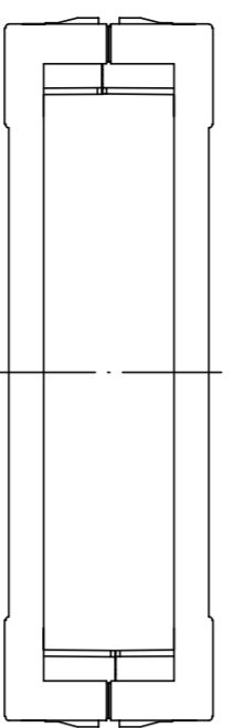
BO 32006 / BO 32009 L (Halbschale niedrig/niedrig) BO 32006 / BO 32009 L (half shell low/low)
